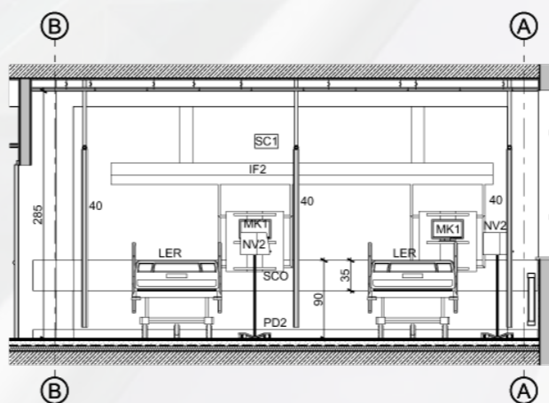
1.58 WST. INT. TERAPIA 03 1:50
