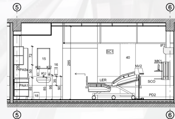
1.58 WST. INT. TERAPIA 02 1:50
