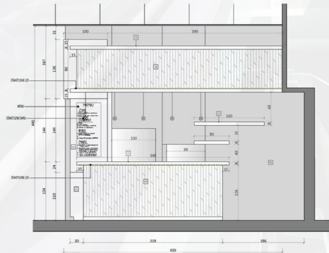
BAR - WIDOK 2 skala 1:25
