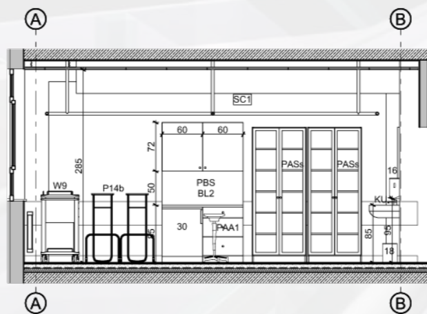
1.58 WST. INT. TERAPIA 01 1:50
