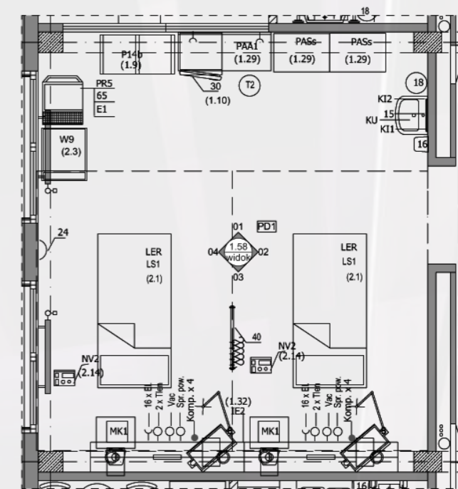
1.58 WST. INT. TERAPIA 1:50
