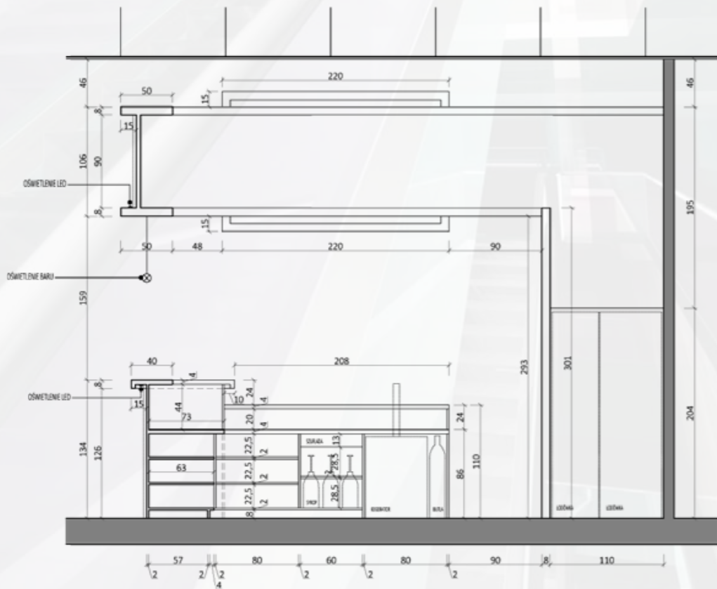
BAR - PRZEKRÓJ C skala 1:25
