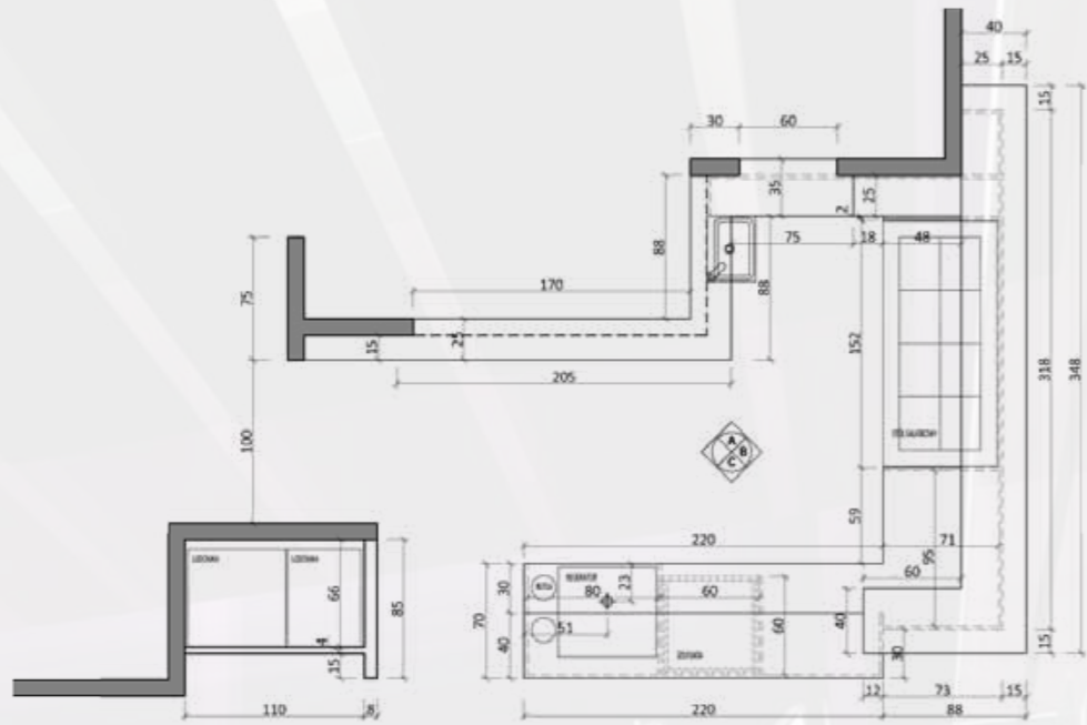
BAR - RZUT 1 skala 1:25
