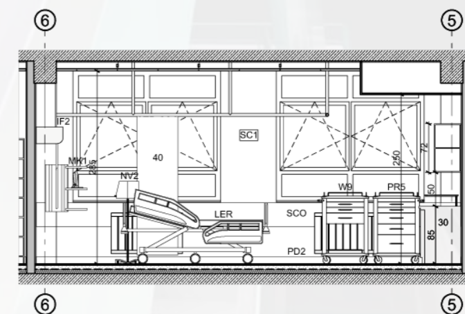
1.58 WST. INT. TERAPIA 04 1:50
